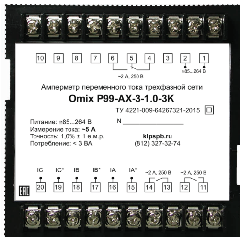
Рис. 7 – Задняя панель прибора
