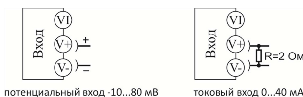
Рисунок 7 – Схема подключения датчиков с масштабированной индикацией
