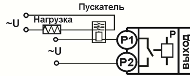
Подключение нагрузки мощностью более 1,5 кВт с помощью электромагнитного пускателя
