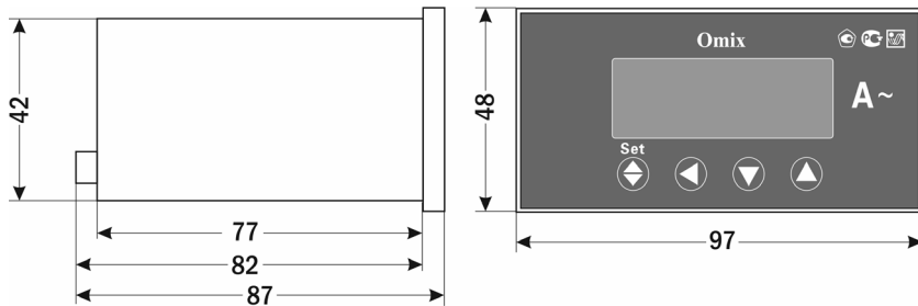
Рис. 5 – Размеры. Тип корпуса P94
