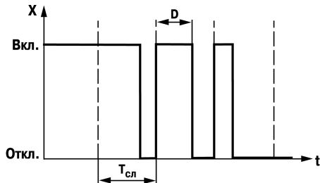
Рисунок 7.11 – Временная диаграмма выходного сигнала ПИД-регулятора
