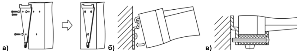
Рисунок 5.1 Монтаж прибора настенного исполнения Н
