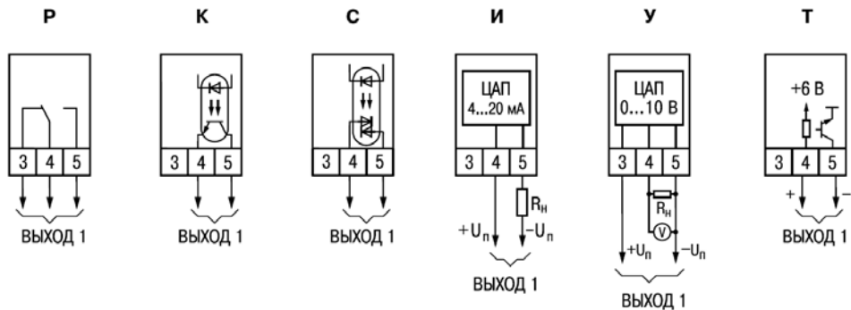
Рисунок В.3 –Схемы подключения различных модификаций выходного устройства 1
