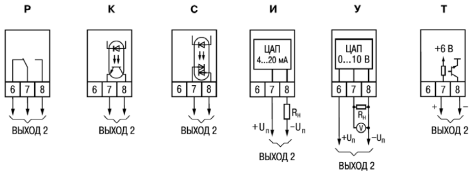
Рисунок В.4 –Схемы подключения различных модификаций выходного устройства 2
