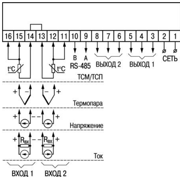
Рисунок В.2 – Общая схема подключения TRM202-H2
