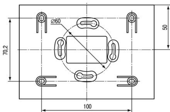
Рисунок А.2 - Прибор настенного крепления Н2
