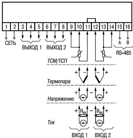
Рисунок В.1 – Общая схема подключения ТРМ202-Н, -Щ1 и -Щ2
