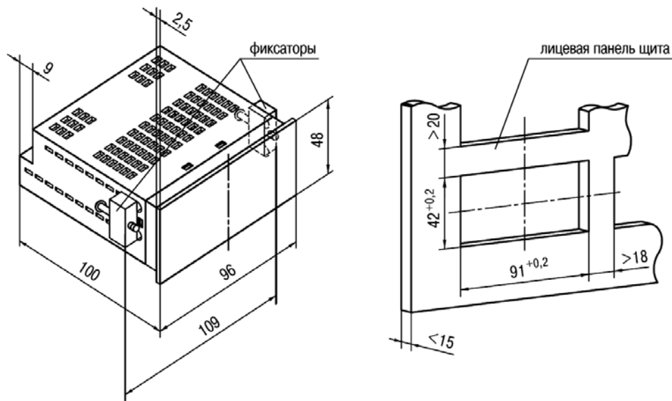
Рисунок А.4 – Прибор щитового крепления Щ2
